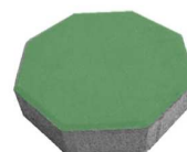
Gạch bát giác (240 x 240 x 60)
